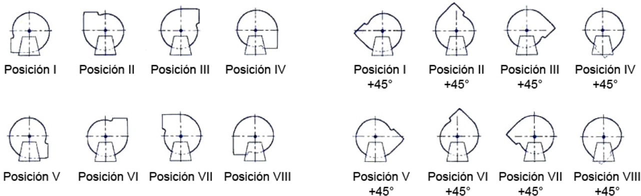
Sentido de giro y Boca de impulsión. Visto lado motor
